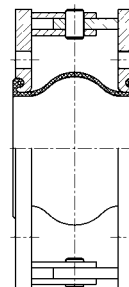
Typ A S klouby, pro úhlový posuv v jedné rovině.
